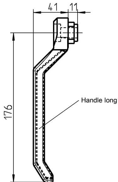
Handle long
